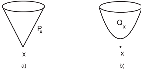
Рис. 5.1: а) связный конический порядок; б) несвязный порядок.
