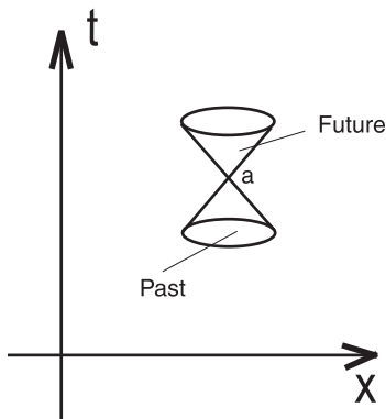
Рис. 1.1: Световой конус в Мире Минковского.
