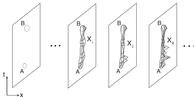
Рис. 14.1: Взаимодействие (неатомарных) событий A и B в плоском Мире Минковского означает наличие материи, соединяющей 4-мерные области A и B в пространстве-времени. Материя – это искривление пространства-времени, изображенное на рисунке в виде горных хребтов X_i , идущих от «горы» A к «горе» B . В действительности мы можем представить себе множество вариантов таких хребтов X_i, X_j, X_k, \dots , включающих «вершины» A и B – пространство-время существует в разных вариантах – Мир многовариантен.
