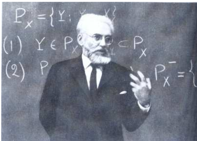
Рис. 12.4: А.Д. Александров: лекция по хроногеометрии.
